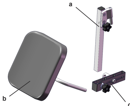
BILD 2. Ingående delar i amputationsbenstöd.
